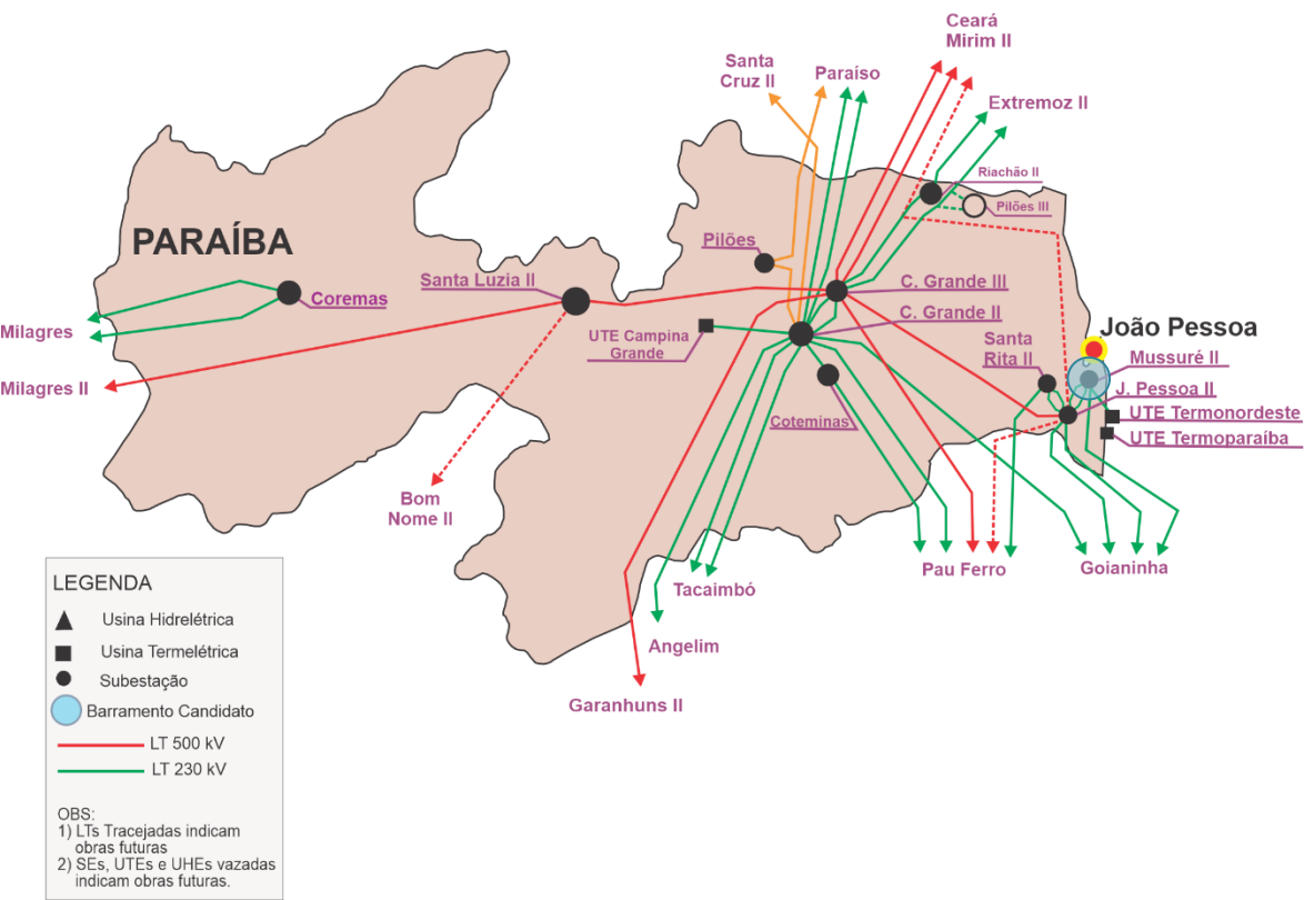
Figura 8-17: Sistema elétrico no estado da Paraíba
