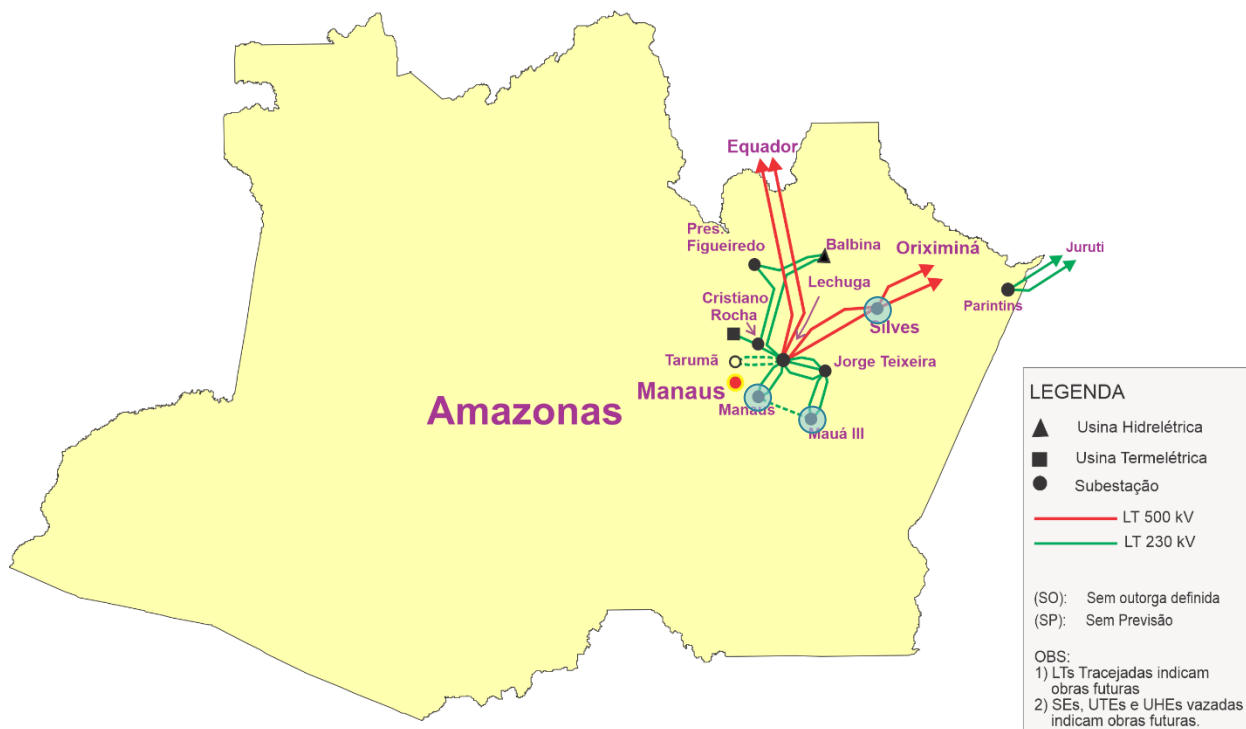
Figura 8-22: Sistema elétrico no estado do Amazonas
